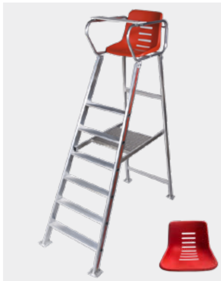
CHAISE DE SURVEILLANCE ALUMINIUM LUXE Réf 7565 : Chaise aluminium luxe avec marches largeur 80 mm renforcées en sous face. Légère et très stable.
